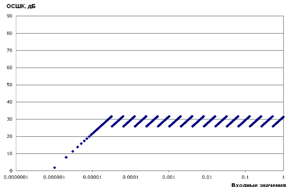
Рисунок 9 – ОСШК для представления с плавающей запятой вида 1–4–5
